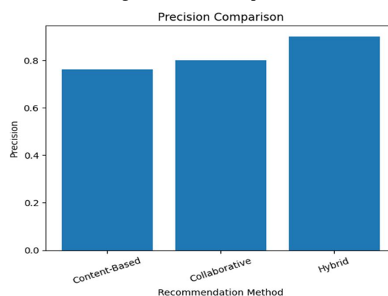
Fig. 4 Precision Graph
