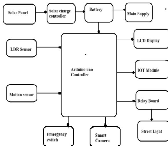
Fig. 1. BlockDiagramofsystem
