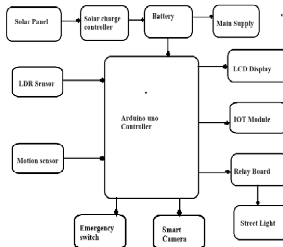
Fig. 1. BlockDiagramofsystem
