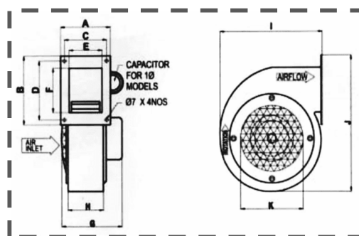
Fig : 8 : Air Blower Design
