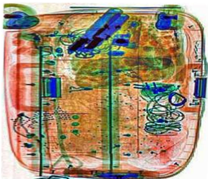
Fig 3. CLAHE
