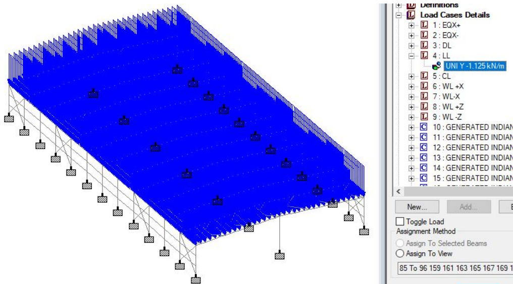
Figure14: Live Load
