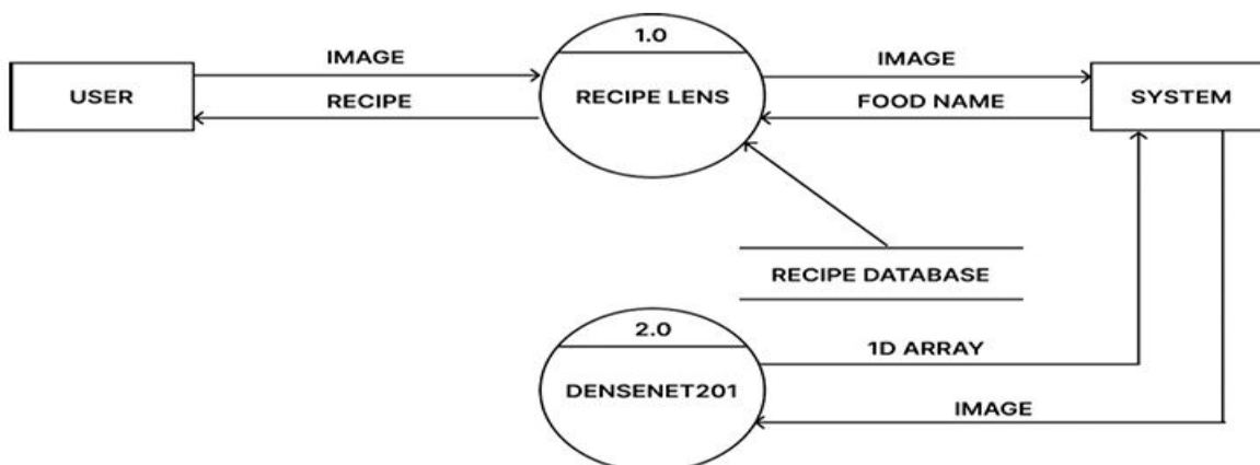
Fig. 3 Level 1 DFD
