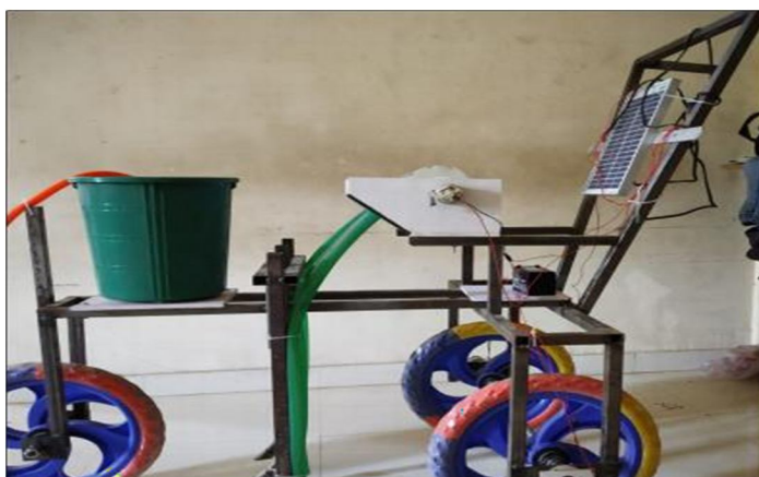
Fig.3: Actual model
