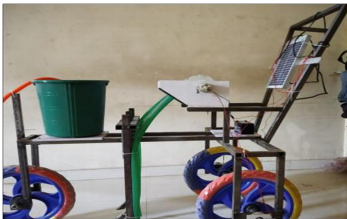
Fig.3: Actual model
