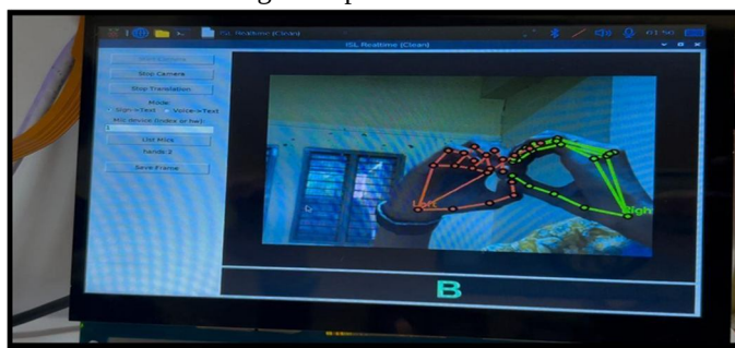
Fig. 2. “Sign-to-Text”
