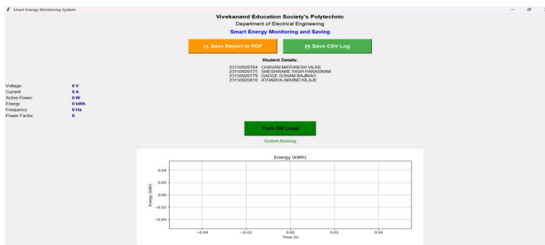
Fig. 3. Python Interface
