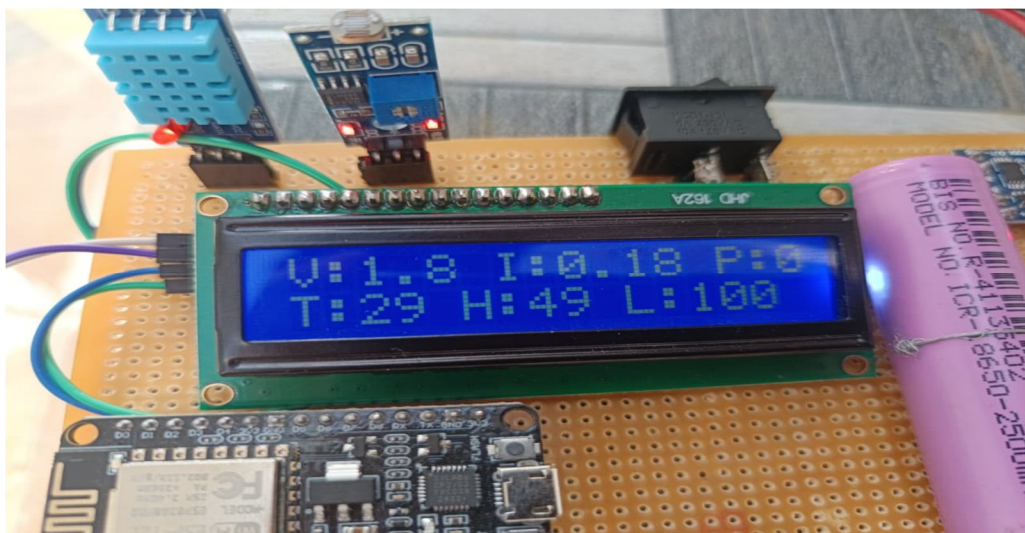
Fig. 4. Real-time parameter readings displayed on the 16x2 LCD
