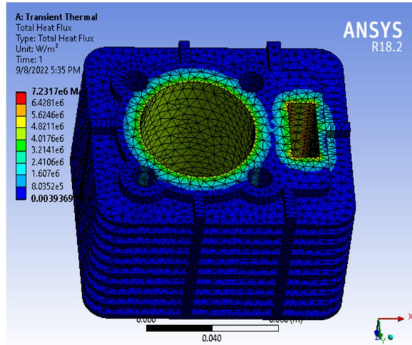
Fig. 12: Fins Al 6061 materials total heat flux at 500°C transient
