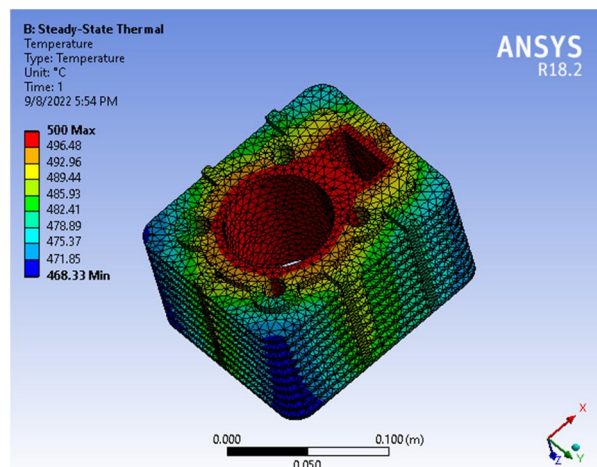
Fig. 15 : Fins Al 6061 materials temperature at 500°C steady
