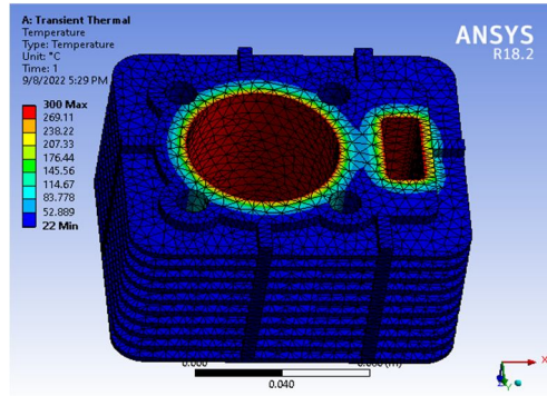
Fig. 8 : Fins Al 6061 materials temperature at 300 0 C transient
