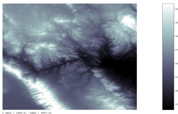
Fig 3: Enhanced DEM
