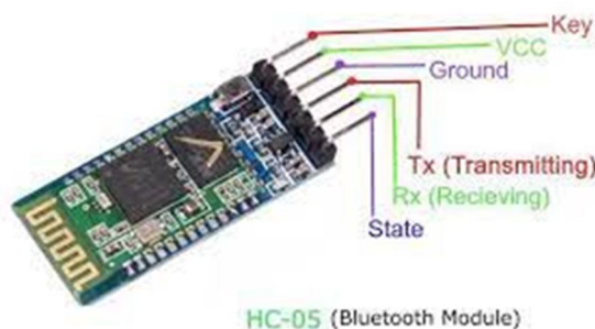
Fig 3 : Bluetooth HC05
