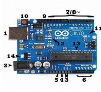
Fig: Arduino Board
